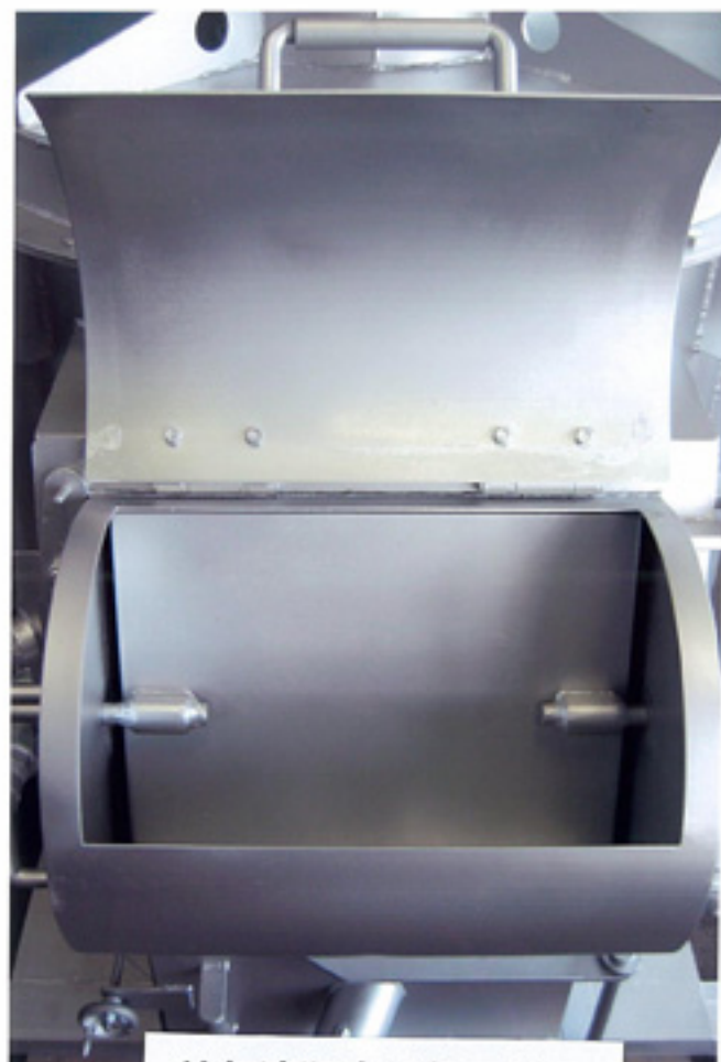
外気遮断定量投入装置 (2ウェイ投入口)
